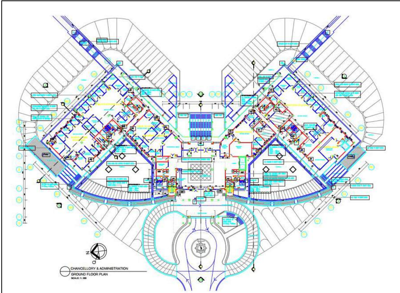
Lakaran pelan kedudukan Galeri Tuanku Canselor UniSHAMS di Dewan Tuanku Permaisuri Hajah Haminah, Kuala Ketil.
